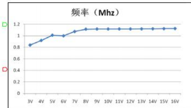
Freq VS Vin
