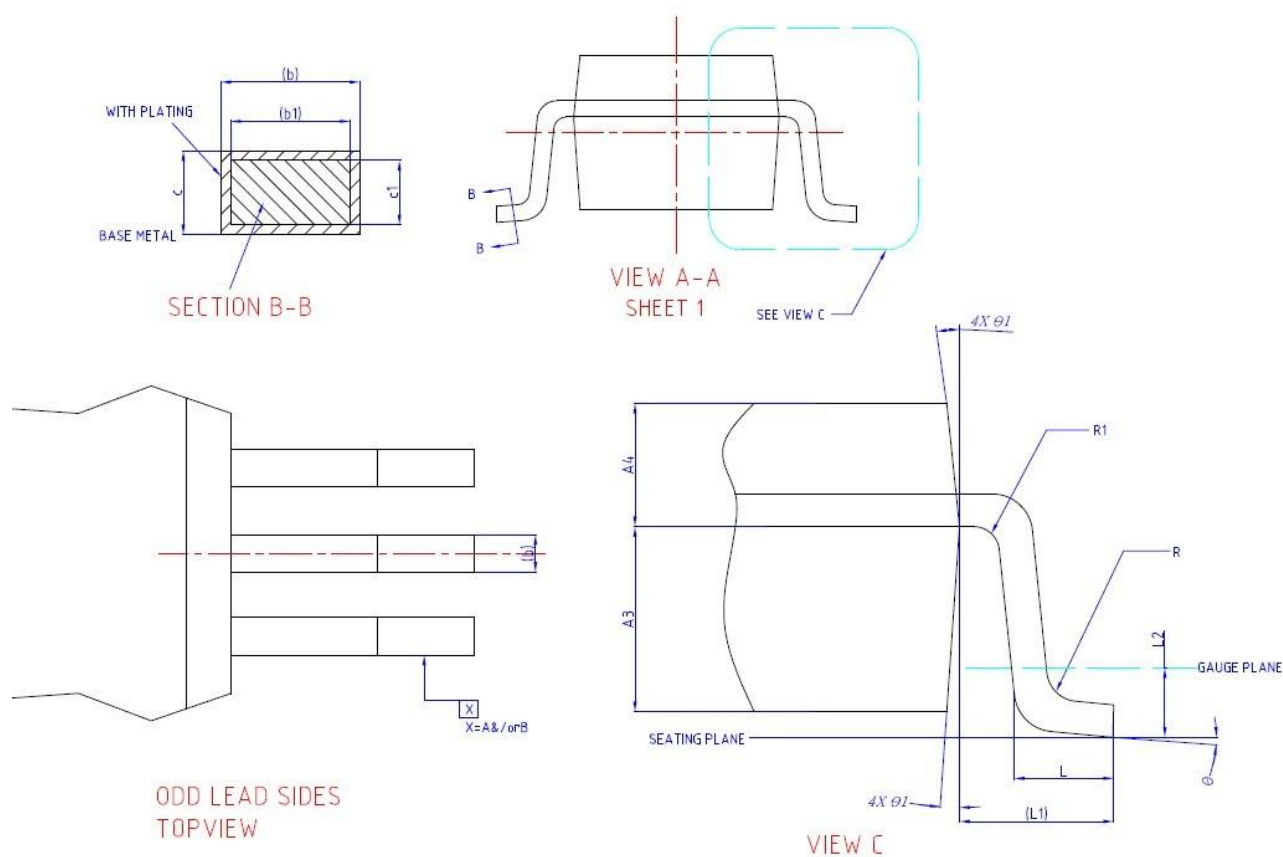
图 3 SOT23-6封装图
